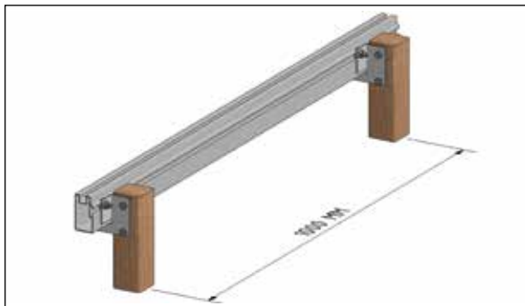
Balk hoog hart op hart afstand 1.000 mm
